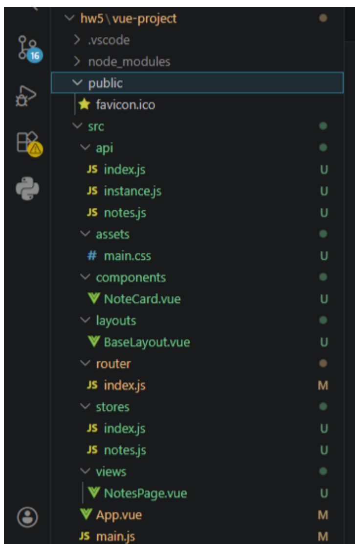
Рис.1. Структура проекта
