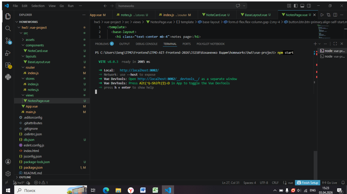
Рис.2. Запуск приложения
